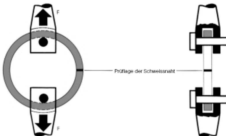
Bild 8: Ringzugversuch
