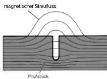
Bild 16: Prüfung mittels magnetischen Streuflusses
