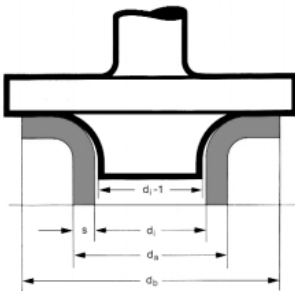
Bild 9: Bördelversuch
