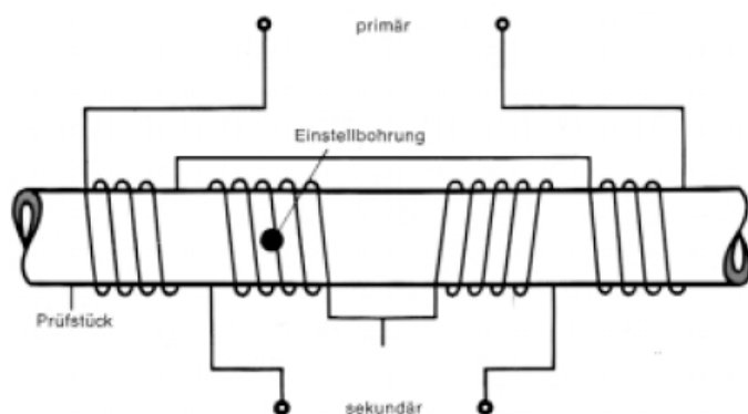
Bild 14: Durchlaufspulen-Selbstvergleichs-Wirbelstromverfahren
