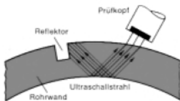
Bild 11: Ultraschallprüfung
