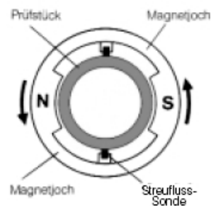
Bild 17: Magnetisches Streuflussverfahren mit rotierenden Magnetisierungsjochen
