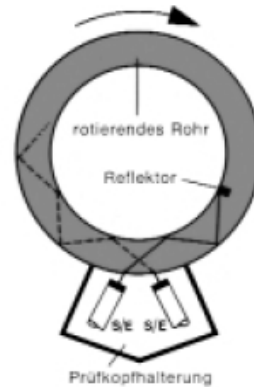
Bild 12: Ultraschallprüfung mit feststehenden Prüfköpfen und rotierendem Rohr
