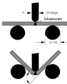
Bild 10: Biegeversuch
