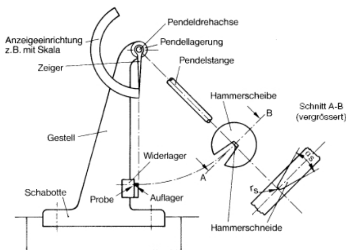
Bild 1: Pendelschlagwerk, schematisch
