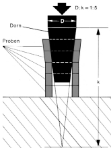
Bild 7: Ringaufdornversuch
