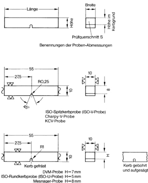
Bild 3: Benennung und Masse der Kerbschlagbiegeproben
