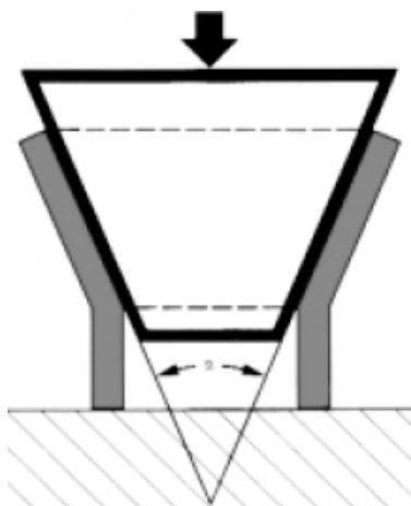
Bild 5: Aufweitversuch
