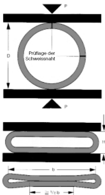
Bild 6: Ringfaltversuch
