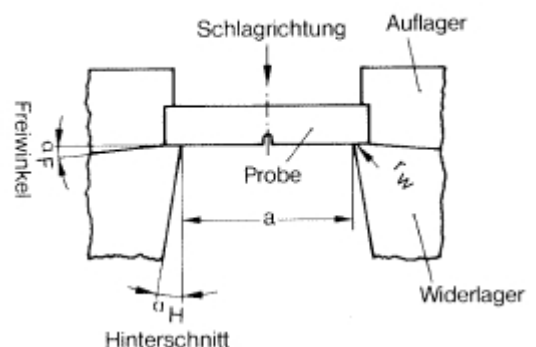
Bild 2: Widerlager und Auflager
