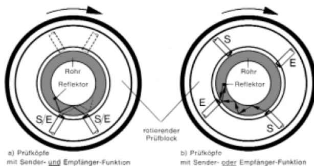
Bild 13a und 13b: Ultraschallprüfung mittels rotierender Prüfköpfe und axial durchlaufendem Rohr
