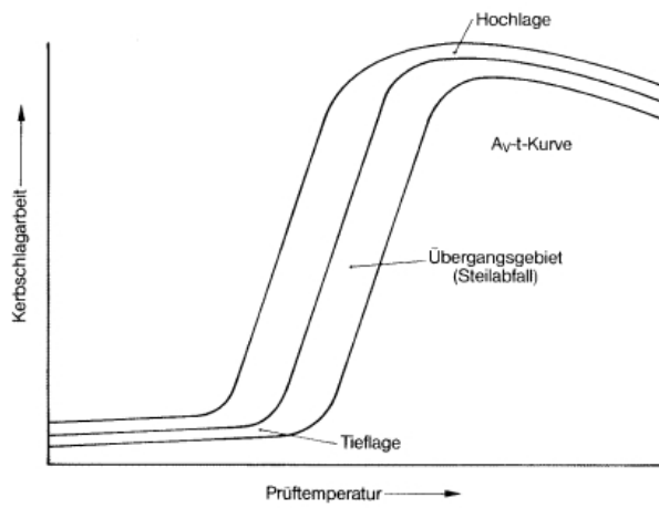
Bild 4: Kerbschlagarbeit-Temperatur-Kurve mit Streufeld
